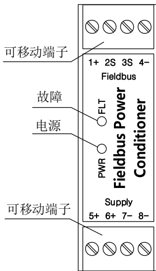
图 2.2 总线电源面板示意图
